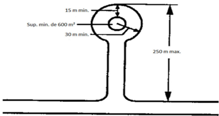
Figure 5: Exemple de dimensionnement de rue en impasse
