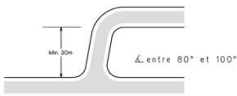
Figure 2: Géométrie des intersections
