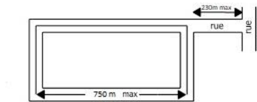
Figure 6: Exemple de rue en tête-de-pipe
